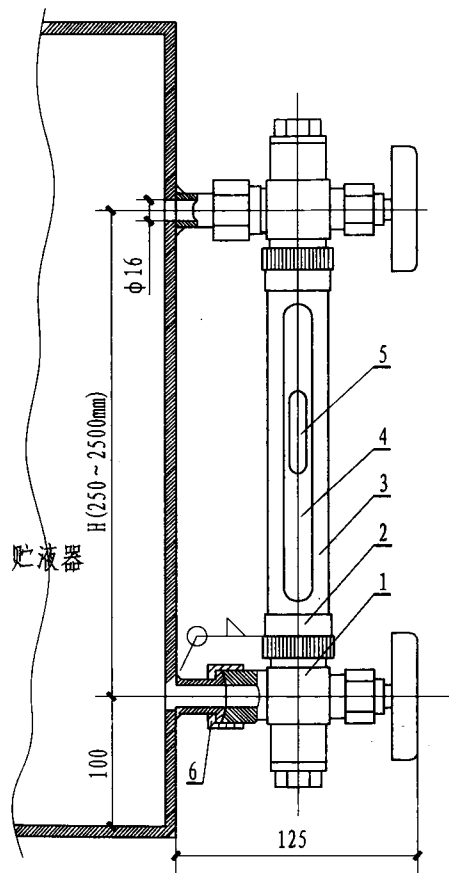
外形图
