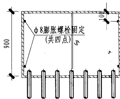
立式水表箱
