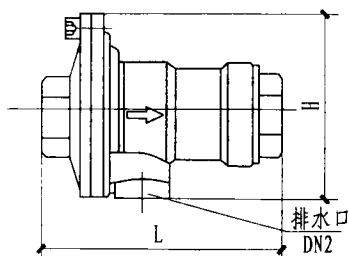
LHS711X型外形
