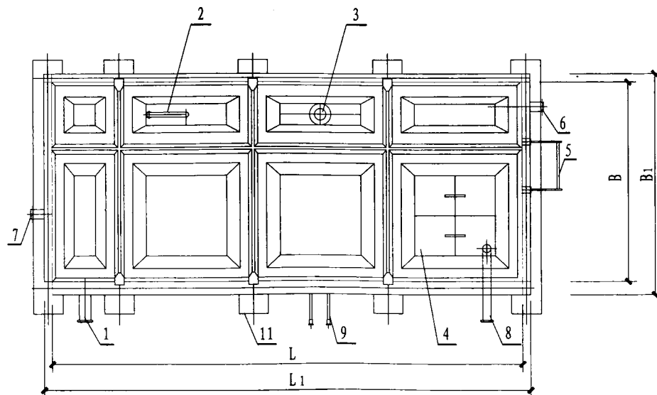
平面图
