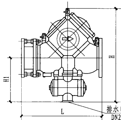
LHS745X型外形
