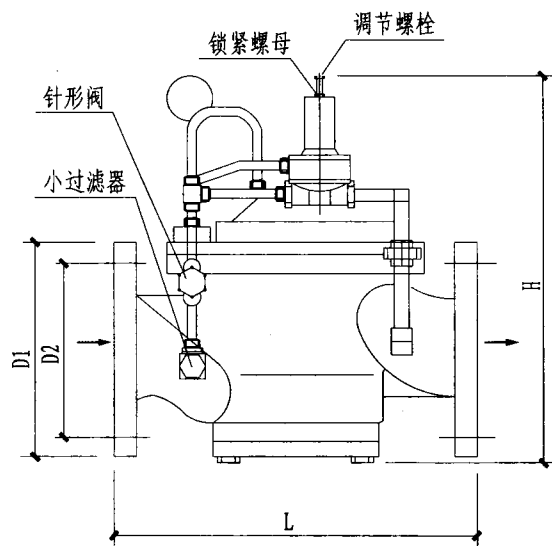
阀体外形图
