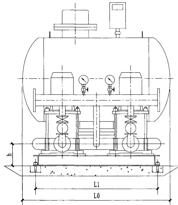
AKK型叠压给水设备(两台泵)立面图
