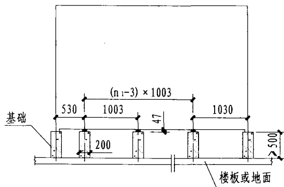
A-A剖面图
