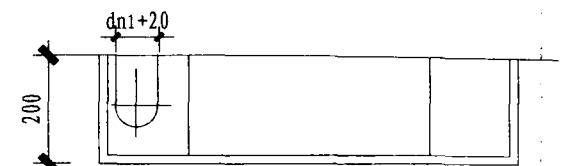
卧式水表箱平面
