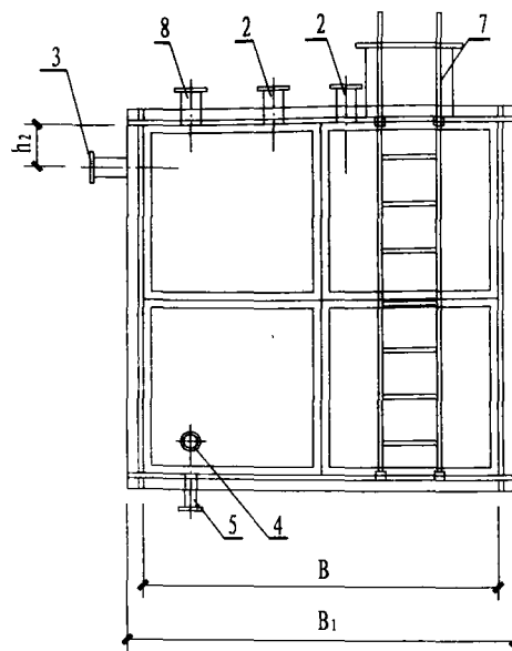
侧立面图
