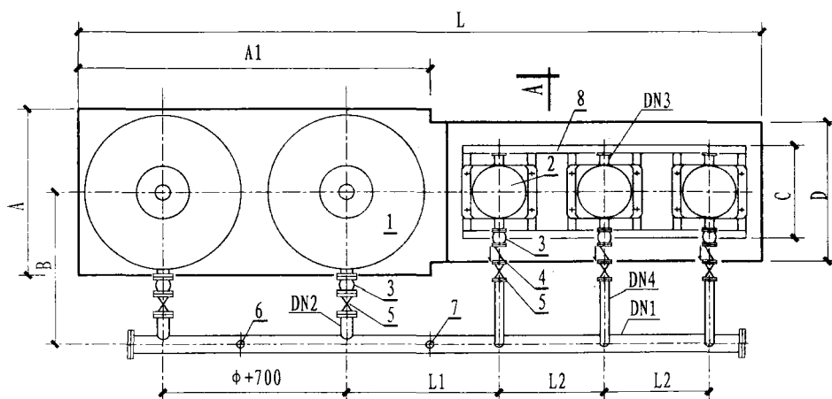
三泵两罐安装图
