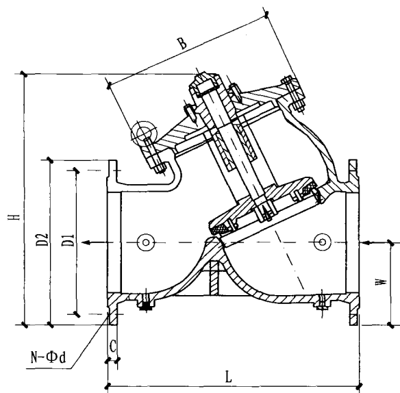
阀体外形图
