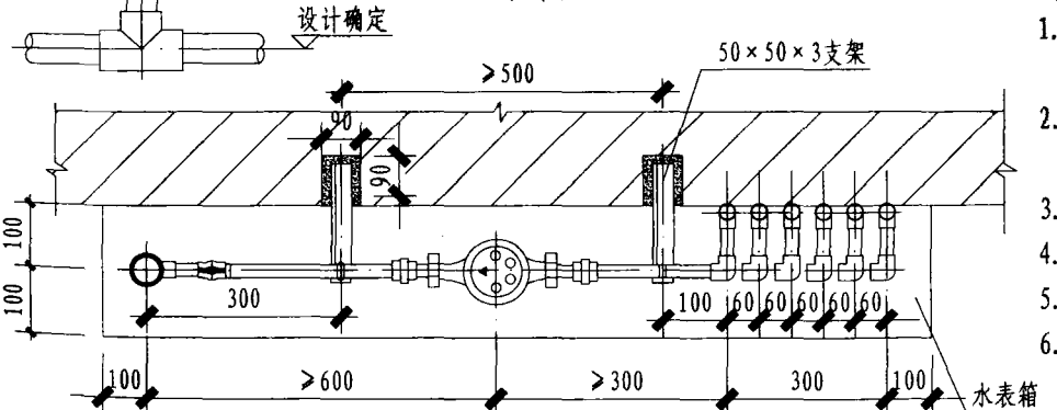
平面图
