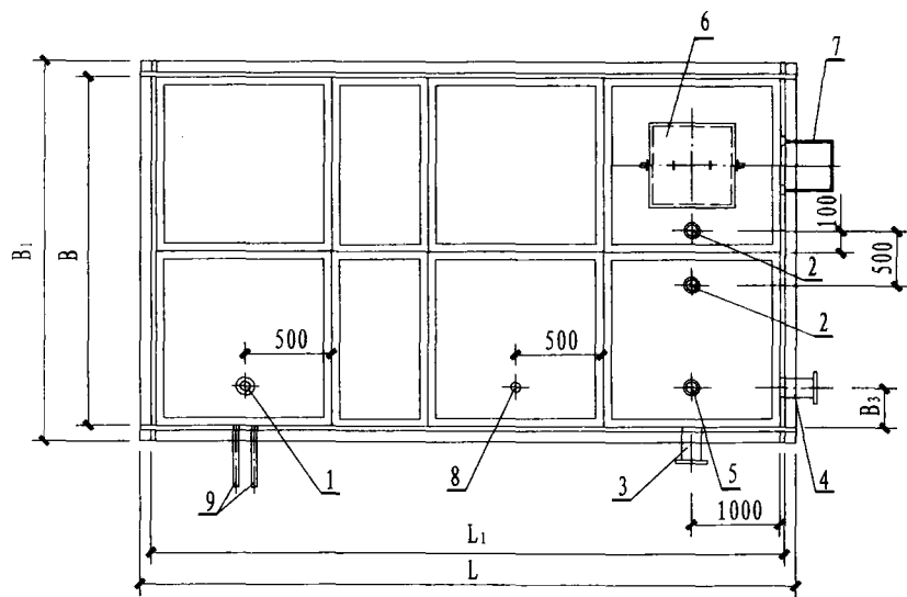
平面图
