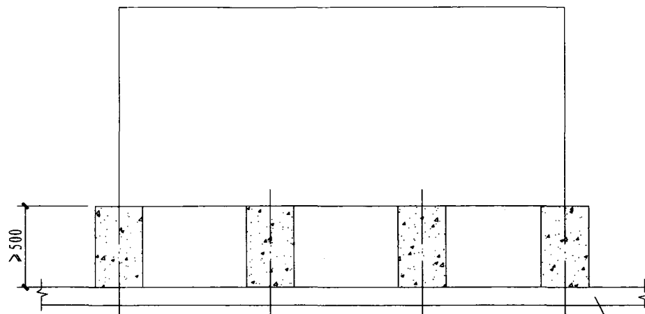
A-A 剖面图
