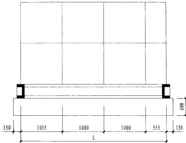
A-A 剖面图
