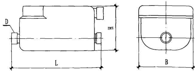
立面图
