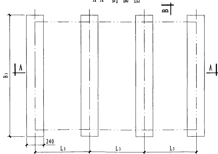
平面图
