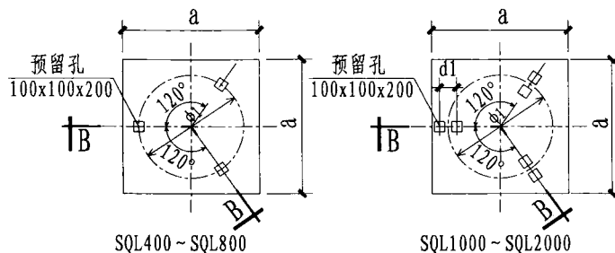
SQL-立式气压罐基础尺寸图
