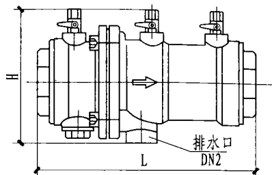
LHS712X型外形
