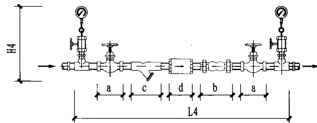
单阀水平安装图
