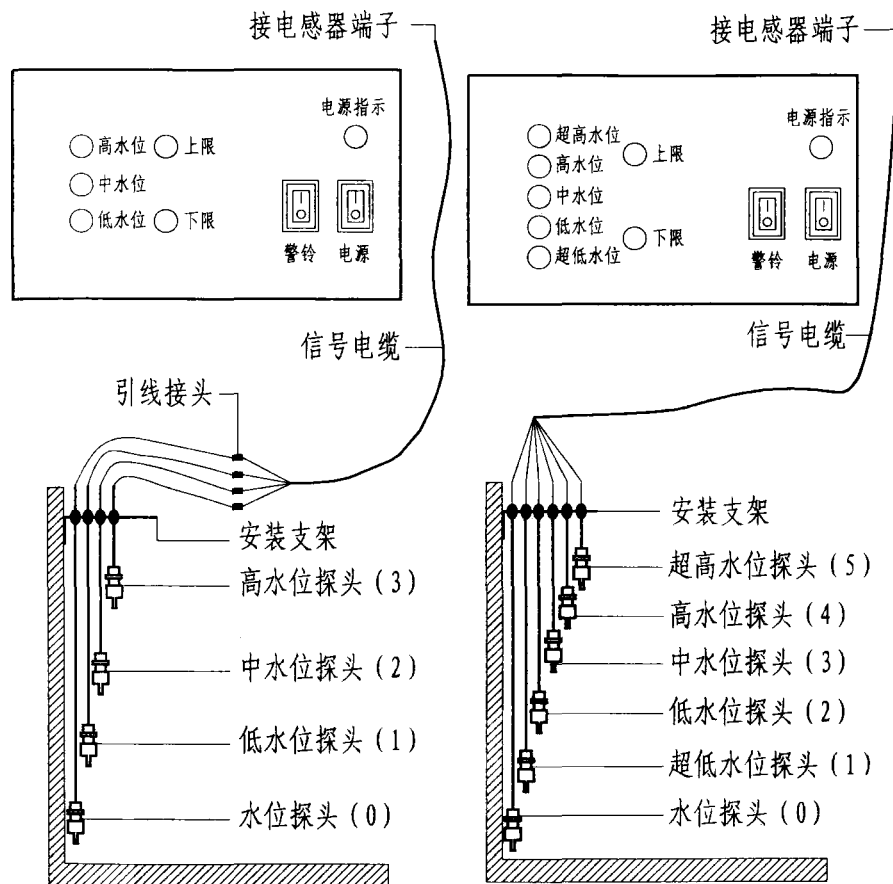
三点式液位控制器接线图
