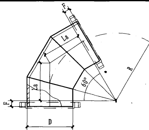
60° 弯头大样图
