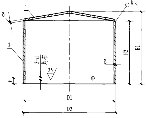
外罩图
