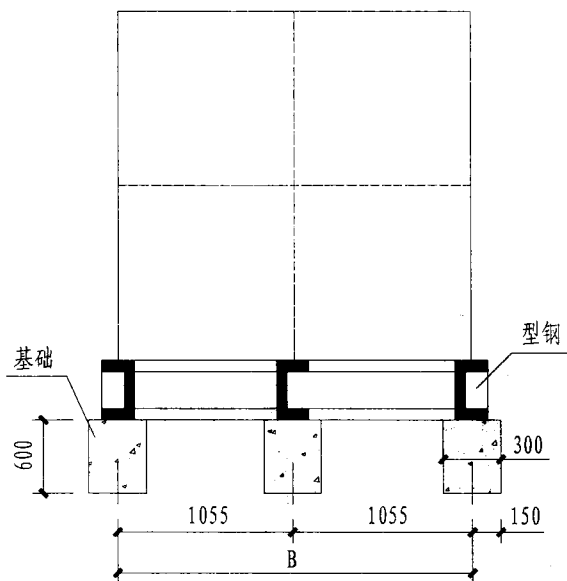
B-B 剖面图
