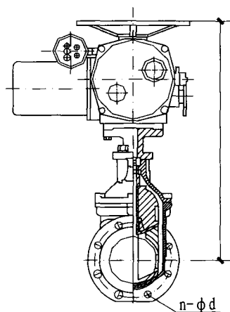
阀体外形图
