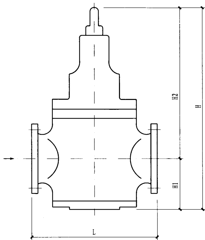
阀体外形图
