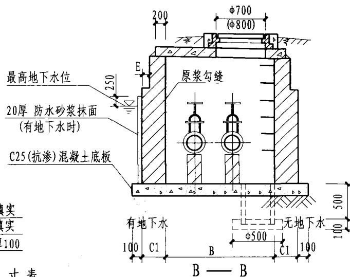
尺寸表
