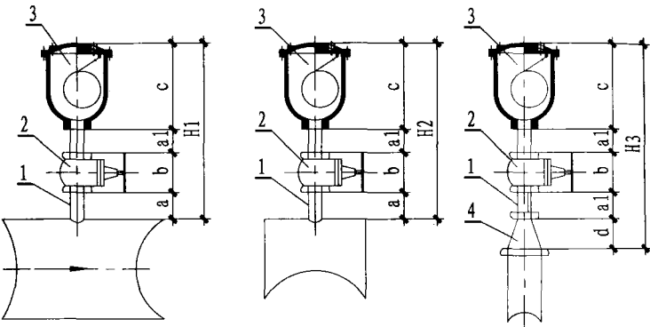
微量排气阀甲型安装
