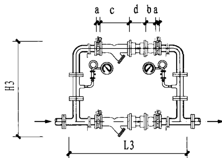
双阀水平安装图
