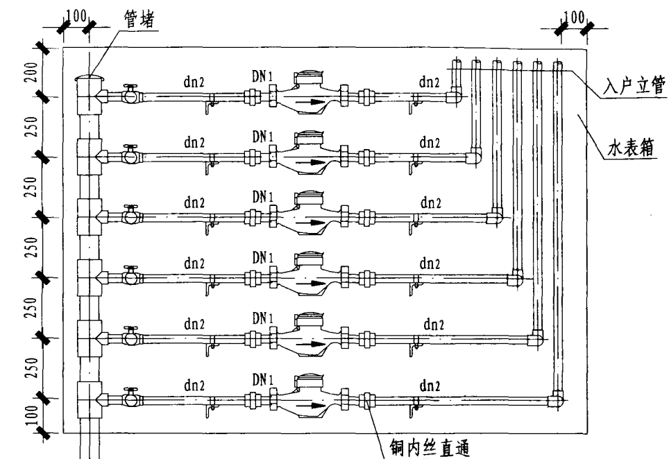
立面图
