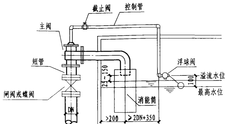
安装示意图
