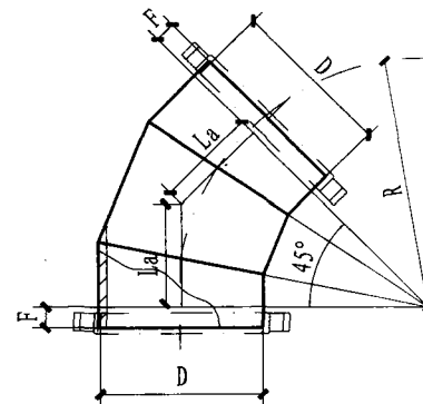
45° 弯头大样图
