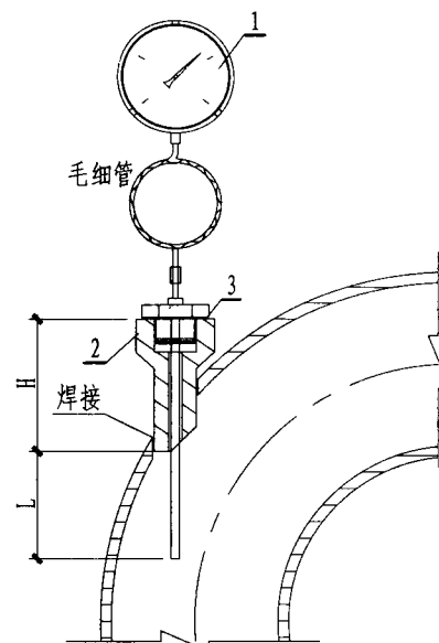
戊型
