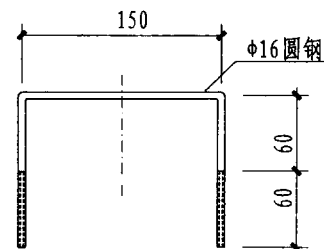
把手大样图
